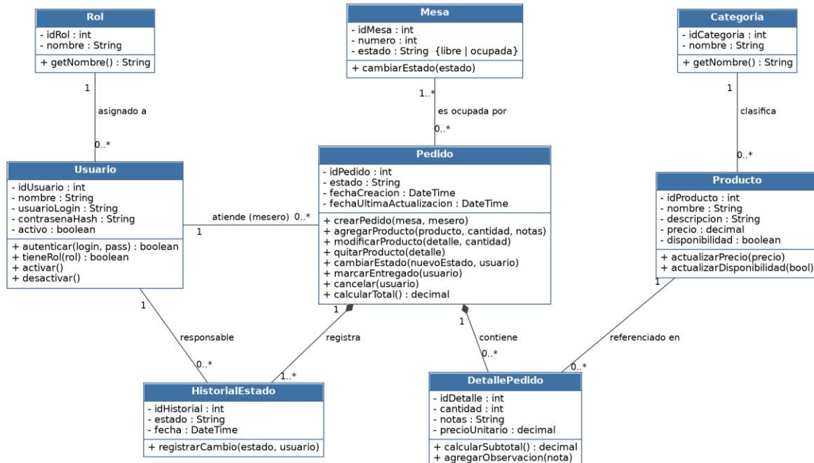
Diagrama de clases — Polirestaurante
